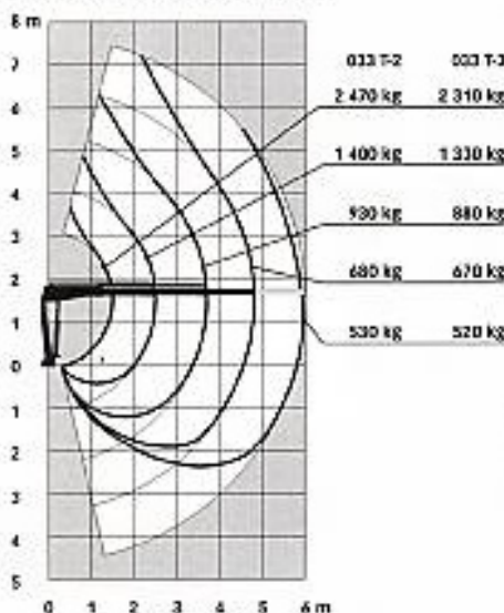
Der HIAB 033 T erfordert auf der Pritsche minimal Platz. Seine niedrige Bauhöhe ermöglicht die Unterbringung unter den meisten Planenaufbauten.
