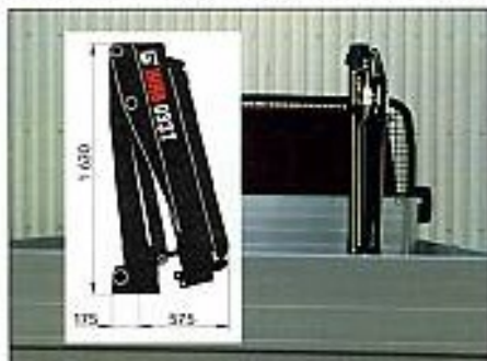
Der HIAB 033 T erfordert auf der Pritsche minimal Platz. Seine niedrige Bauhöhe ermöglicht die Unterbringung unter den meisten Planenaufbauten.
