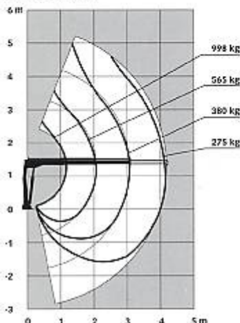
Der HIAB 013 T erfordert auf der Pritsche minimal Platz. Seine niedrige Bauhöhe ermöglicht die Unterbringung unter den meisten Planenaufbauten.
